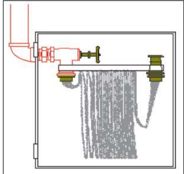
Figura 3 – Suporte para mangueira tipo “rack”
